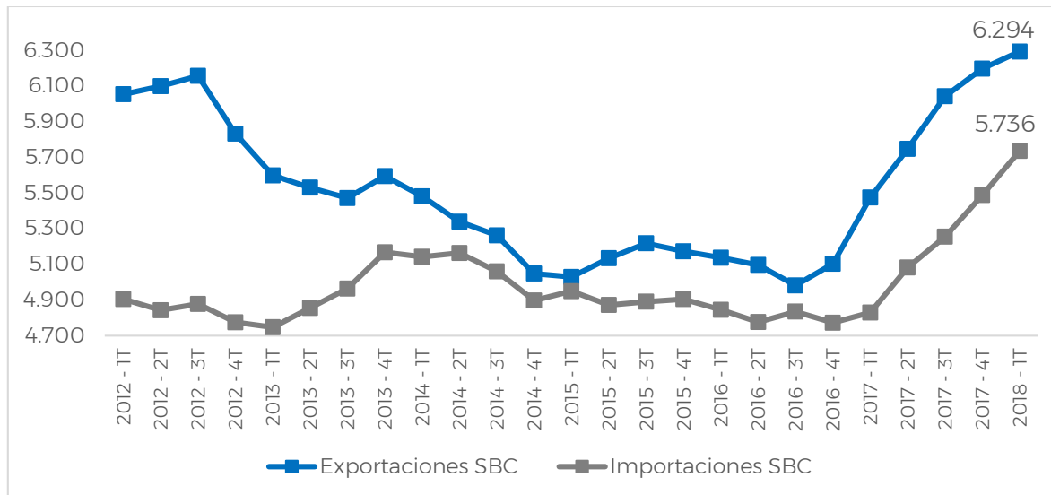
GRÁFICO 1. COMERCIO INTERNACIONAL DE SBC DE ARGENTINA Valores en millones de USD, suma móvil 4 trimestres.
