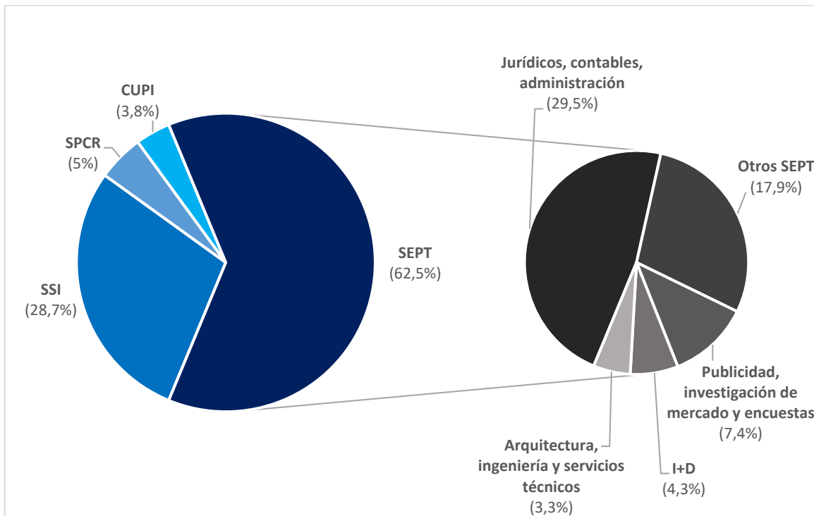
GRÁFICO 2. RELEVANCIA SECTORIAL EN LAS EXPORTACIONES ARGENTINAS DE SBC Porcentaje sobre el total exportado en los últimos 4 trimestres.
